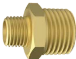
170800 Amarelo Rosca Externa: NPT 1/2" NIPLE DE REDUÇÃO Rosca Externa: NPT 1/4"
