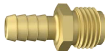
170301 Amarelo TERMINAL TC X TM Saída Externa: TM 3/8" Rosca Externa: TC 1/2"
