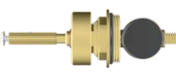
039153 Acabamento: ARGUS Deca Dream, Polo e Level Bitola: 3/4 Estria: Deca Dream Rosca: N° 117 Cunha: N° 70
