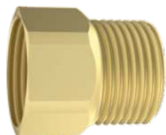
150350 Cromado AUMENTO 15mm 3/4" X 3/4" Rosca Externa: 3/4" Rosca Interna: 3/4" Comprimento: 15mm
