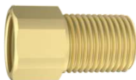
150301 Cromado AUMENTO 25mm 1/2" X 1/2" Rosca Externa: 1/2" Rosca Interna: 1/2" Comprimento: 25mm
