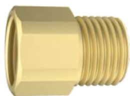
150300 Cromado AUMENTO 15mm 1/2" X 1/2" Rosca Externa: 1/2" Rosca Interna: 1/2" Comprimento: 15mm
